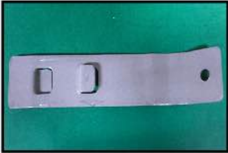
後輪擋泥板 鐵扣 Rear fender bracket
